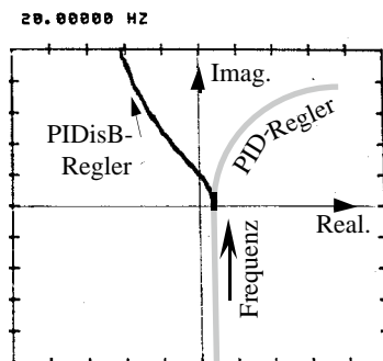
Bild 20: Frequenzgang des PIDisB-Reglers (dargestellt als FFT-Nyquist-Diagramm) gemessen über synchronisiertem Regler inklusive netzgeführtem Stromrichter. (U/E vgl. Bild 14). Bis zu 120 Grad positiver Phase sind daraus abzulesen. Der konventionelle PID-Regler kann dagegen prinzipiell, wie grau skizziert, nur maximal 90 Grad positive Phase aufweisen.
