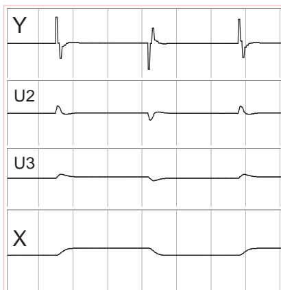
Bild 18: Signalverläufe gemessen im geschlossenen Regelkreis mit 3 Verzögerungen optimiert mit PDisB-Regler (vgl. Bild 16) Die Meßergebnisse Bild 17 bis Bild 19 machen den Vorzug des PDisB bzw. des PIDisB-Reglers gegenüber dem PID-Regler im
